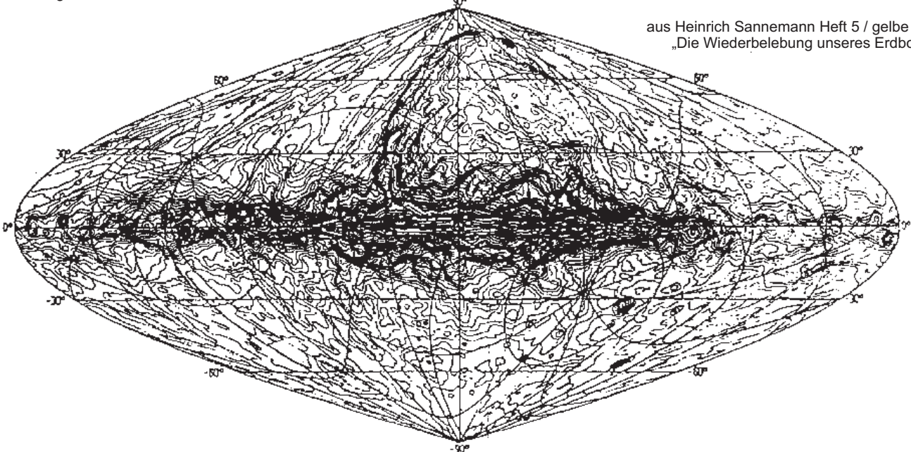
Gesamtansicht des Radiohimmels als Radiokontur-Karte
